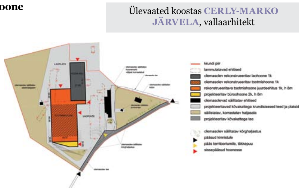
Asendiskeem.
